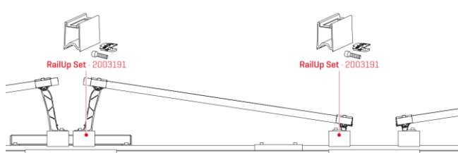
Version D-DOME 6 CLASSIC avec RailUp
